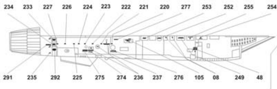
Су-27 всех производственных серий, левый двигатель, внутренняя сторона мотогондолы Su-27 from all productional batches, port side engine, inner surface of engine compartment
