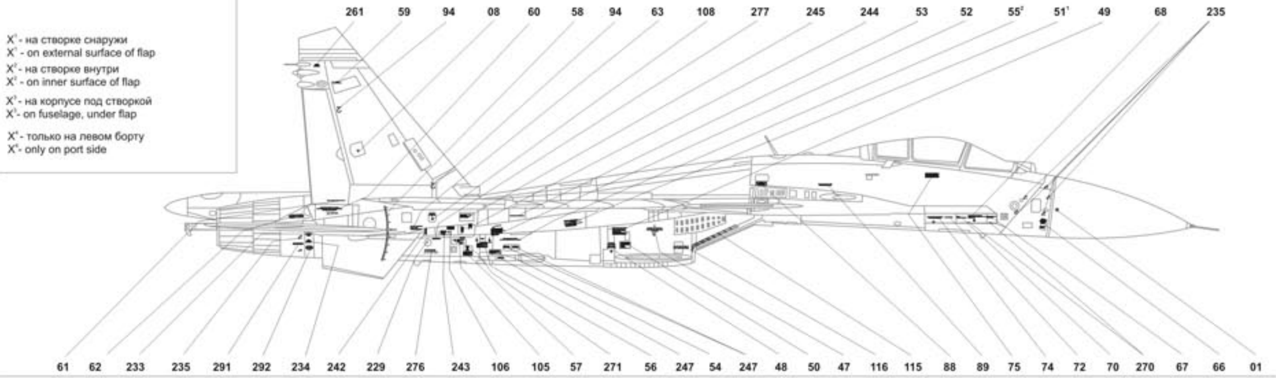
Су-33 4-ой - 9-ой производственных серий, вид слева Su-33 from 4-th to 9-th production batches, port side view
