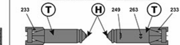
Бомба ОФАБ-250ШН x 10 OFAB-250ShN bomb x 10
