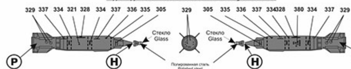
Корректируемая бомба КАБ-500Л x 2 KAB-500L gilded bomb x 2
